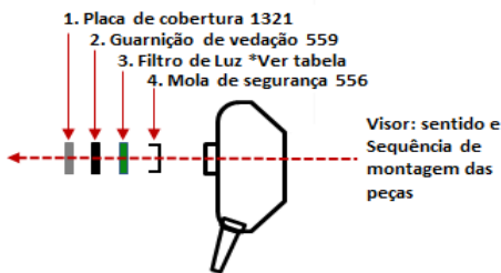
Escudo de solda: Esquema de montagem das peças
