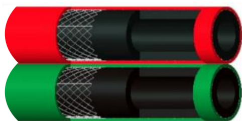
Vista em corte das mangueiras mostrando as camadas da estrutura de montagem
